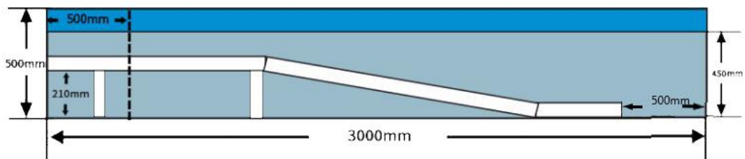
图 4.3.2 (2) 管道检测场地图【侧视图】
