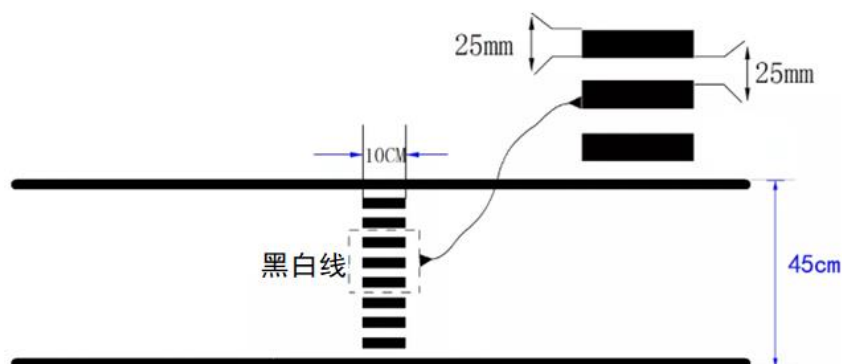
图 7.14 起点/终点示意图
