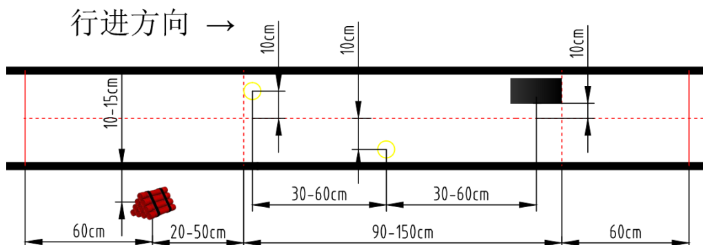
图 7.9 危险区示意图
