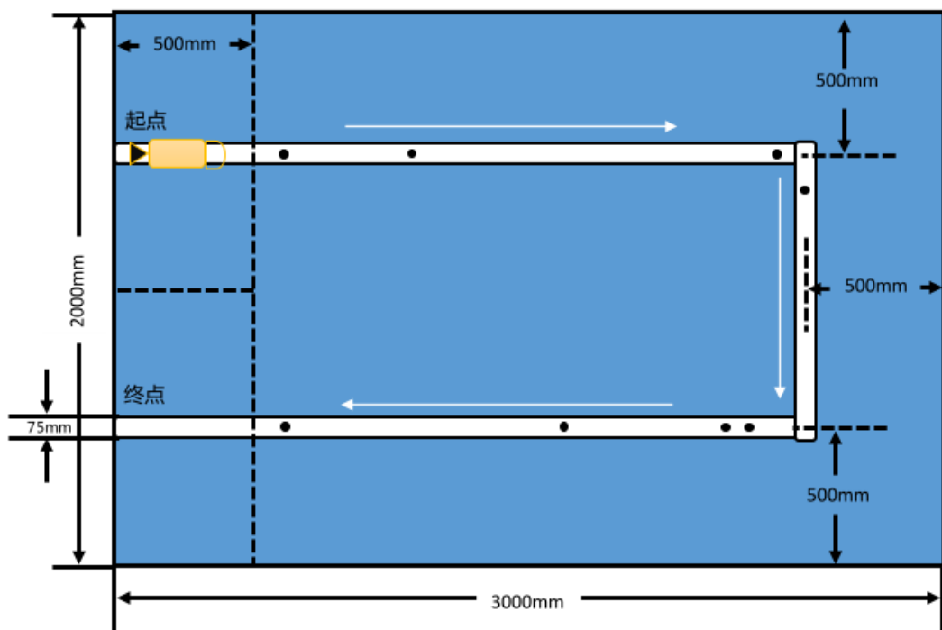
图 4.3.1 (1) 管道检测场地图【俯视图】
