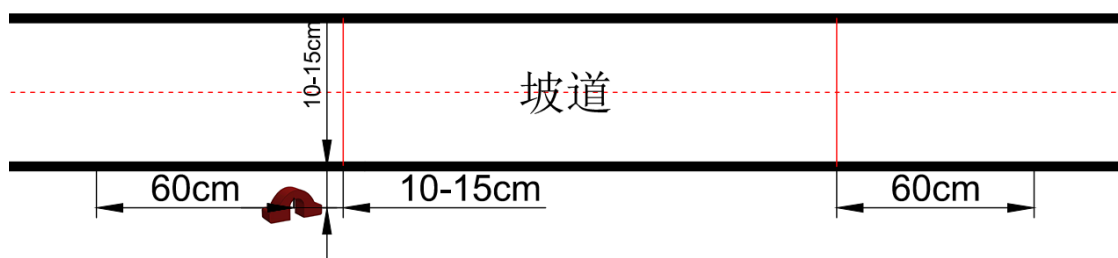
图 7.13 坡道示意图
